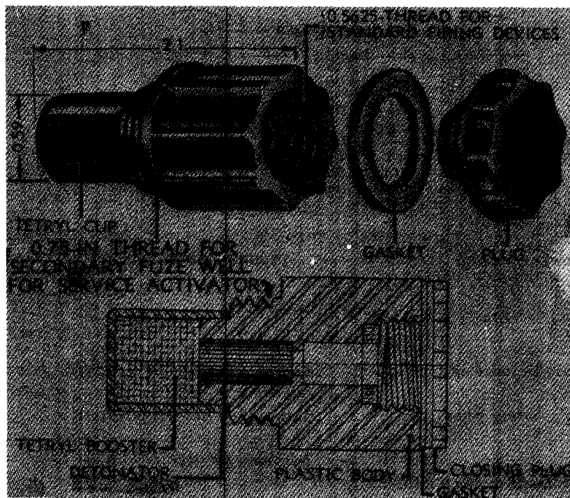
Fig 14 ACTIVATOR M1
